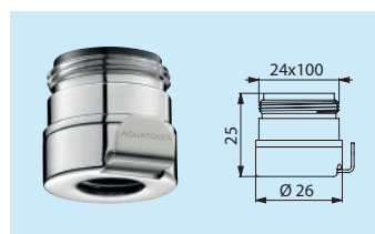
Sortie M24x100
