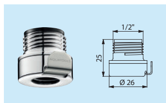
Sortie M1/2"
