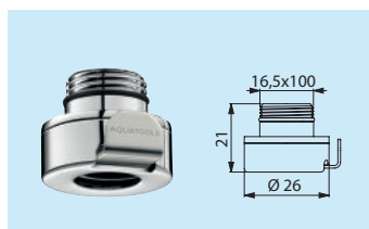
Sortie M16.5x100
