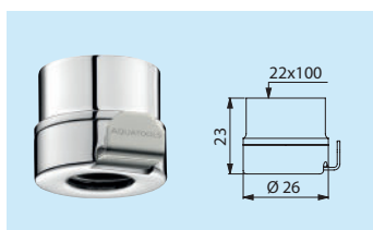
Sortie F22X100
