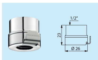
Sortie F1/2"
